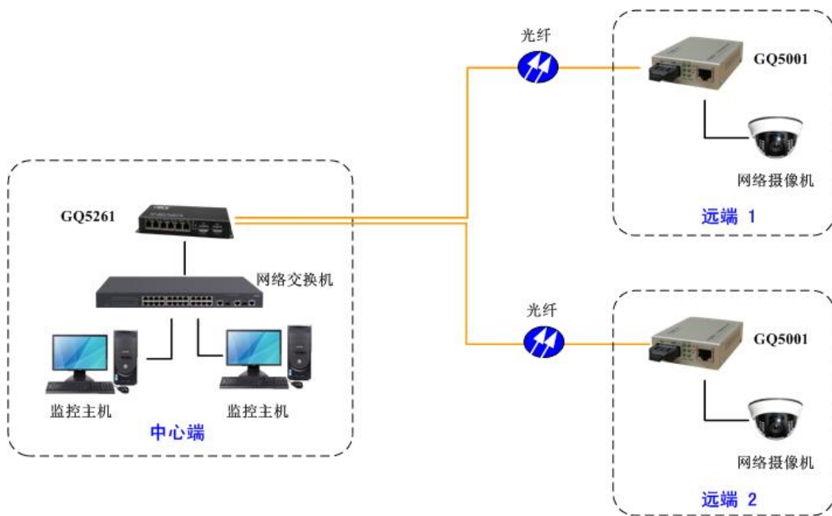
方案二：光纤 1 点对 2 点组网
